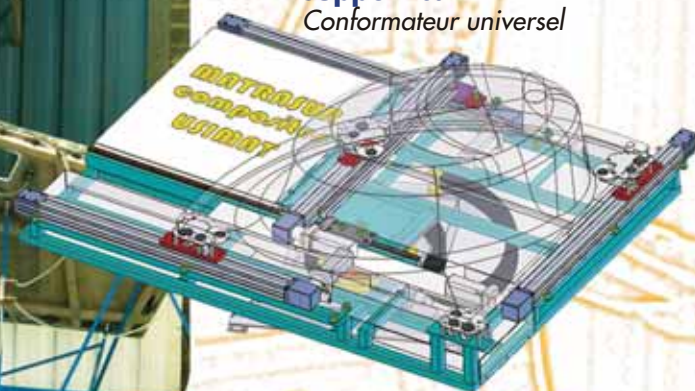
Automatic mould positioning system Indexage automatique chariot conformateur
